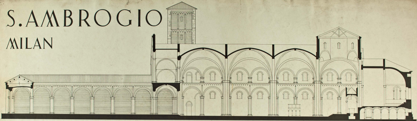
LONGITUDINAL SECTION
