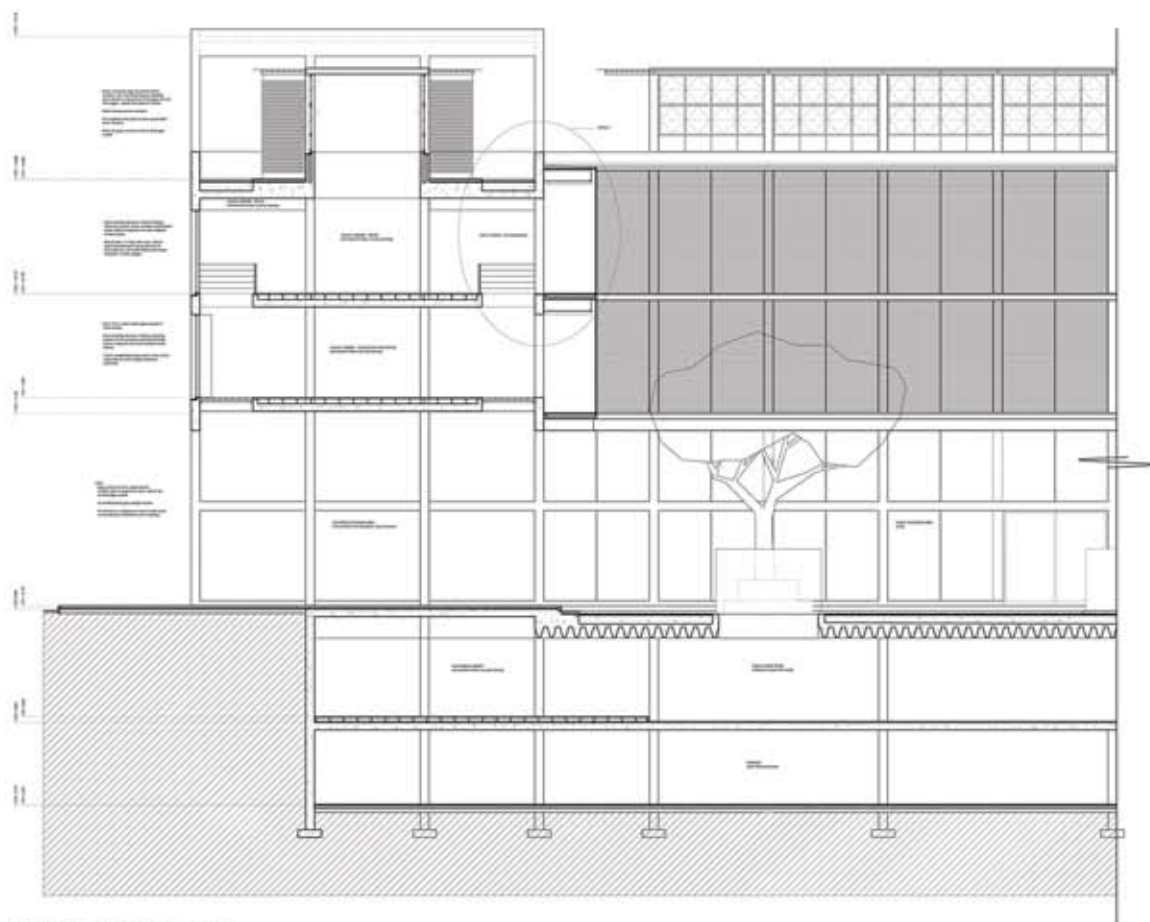
PARTIAL SECTION B-B, N.T.S.
