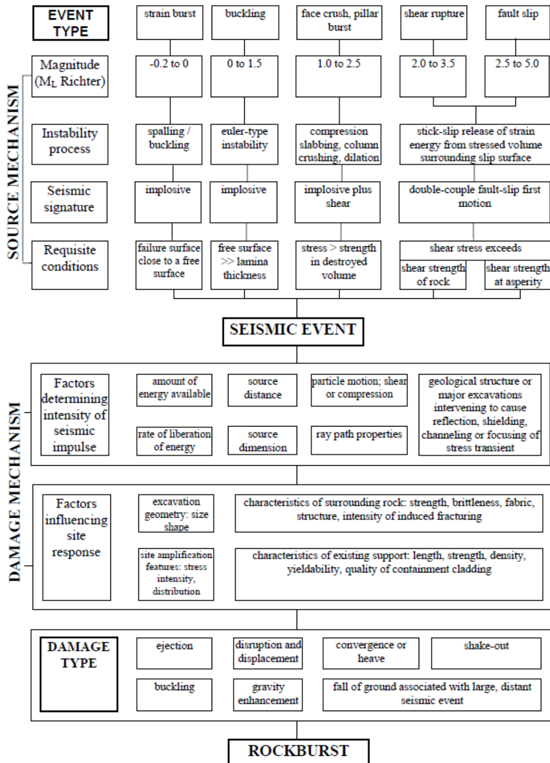
Figure 2-7: Rockburst flow chart (Ortlepp, 1997)
