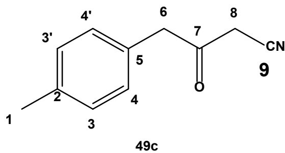
1 H NMR of 49c
