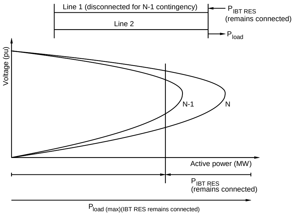
Figure 8 – No IBT RES
