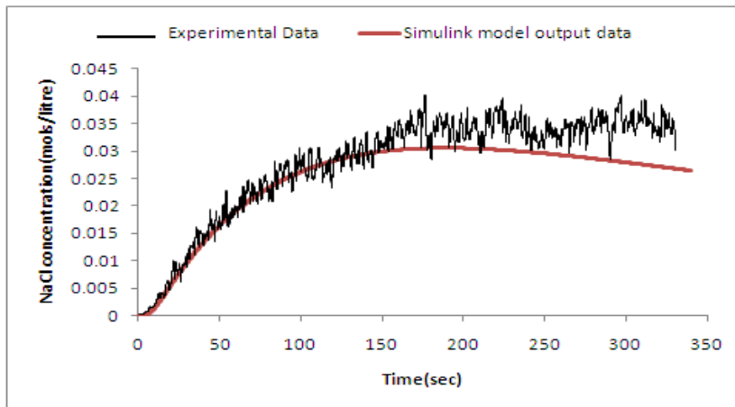
b) 10ppm MIBC 30mm riser
