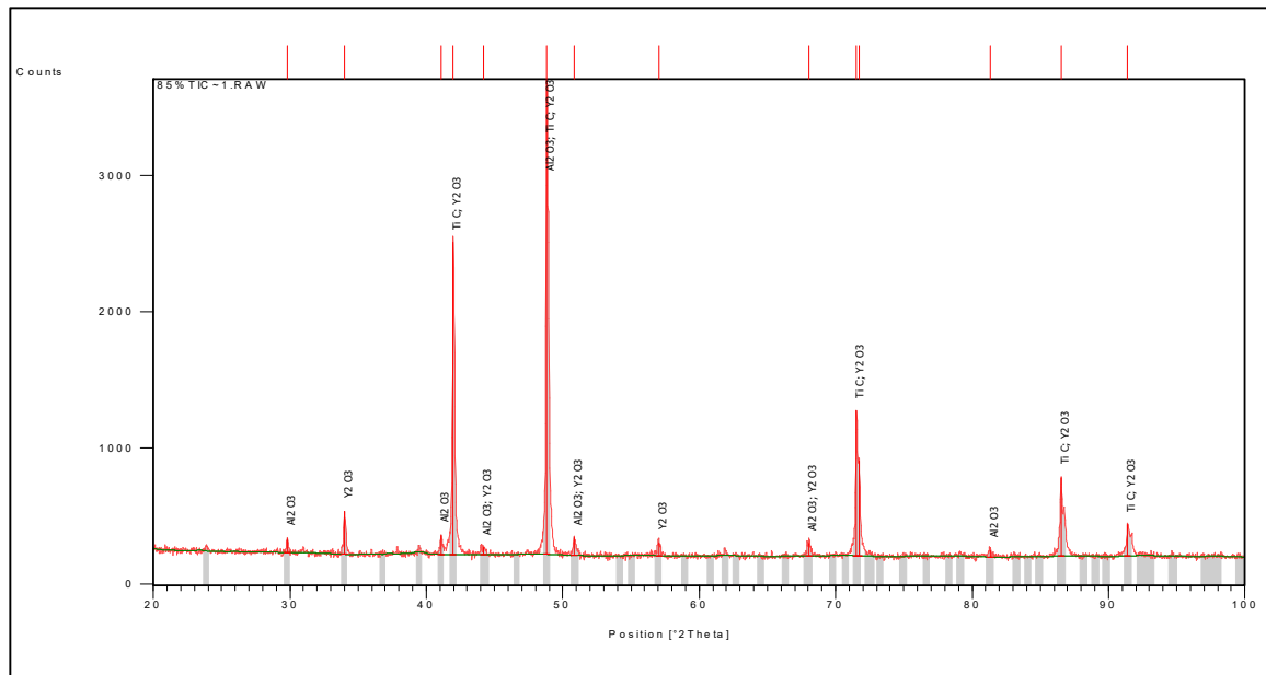
Figure 4.2a) 85 wt. % TiC +12 wt. % Al 2 O 3 + 3 wt. % Y 2 O 3 powder
