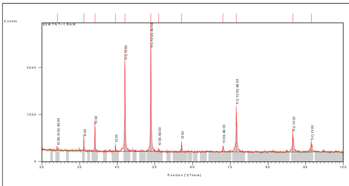
Figure 4.2b) 85 wt. % TiC-3.75 wt. % Al 2 O 3 -6wt. % Y 2 O 3 -5.25 wt. % SiO 2 powder
