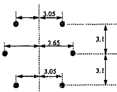
Figure 4.5.1.a: Goudey-Oakdale Line Dimensions
