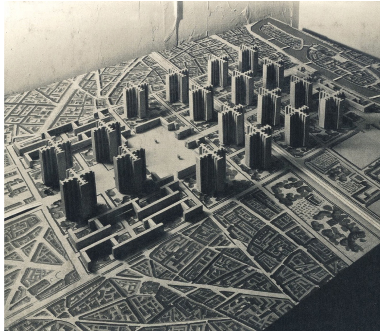
017. Plan Voisin
