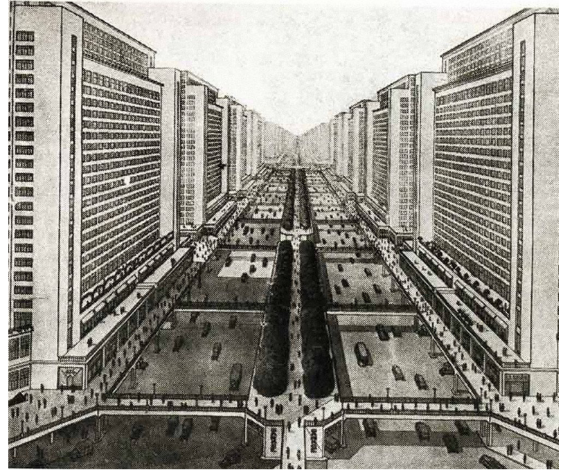
015. Ville Radieuse
