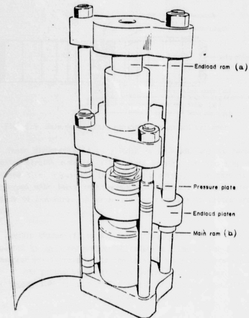
Fig. 3.4 The Kennedy Press
