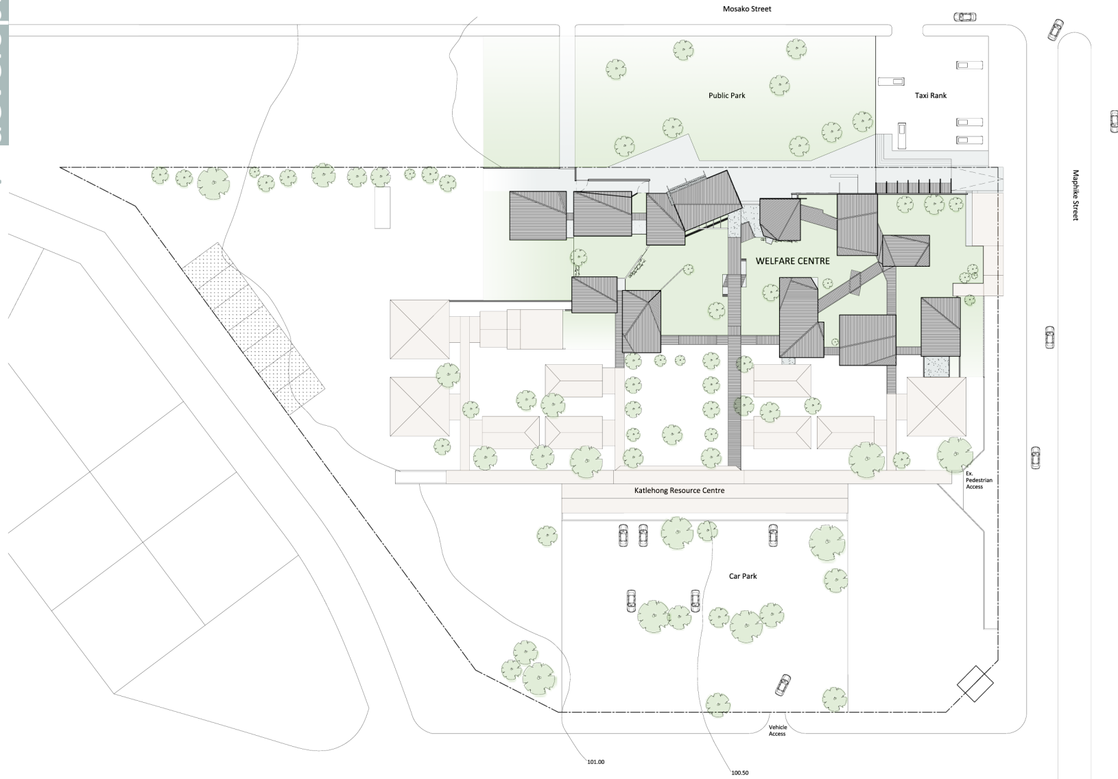
Site Plan 1:1000
