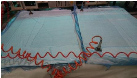
(d) Vacuum bagging
