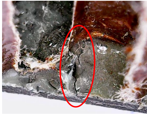
(d) Bond line matrix cracking at CP-A
