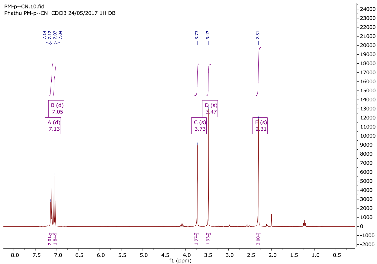
13 C NMR of 49c
