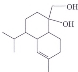
T-cadinol
