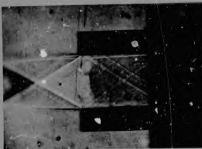
Fig. 56 #2 M2 Schlieren
