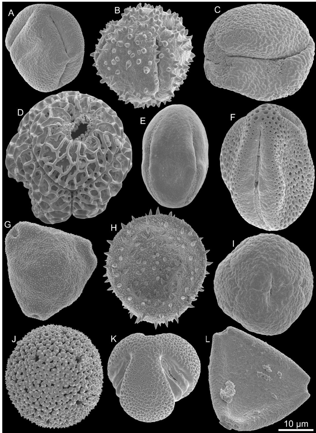
Figure 1. SEM micrographs of fossil pollen from the early Miocene of Saldanha Bay (South Africa). A , Rhizophoraceae. B , Viscaceae. C , Araceae. D , Winteraceae. E , Sapotaceae. F , Vitaceae. G , Casuarinaceae. H , Picrodendraceae. I , Ericaceae. J , Thymelaeaceae. K , Euphorbiaceae. L , Proteaceae.
