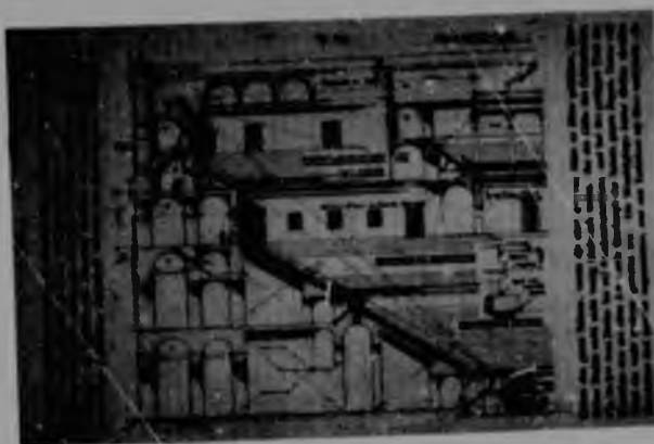
13. Colosseum, Rome, section. Durm, Baukunst der Etrusker und Römer , fig. 745.
