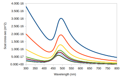
(d) \text{Ag}@/\text{SiO}_2 core-shell NPs scattering cross-section
