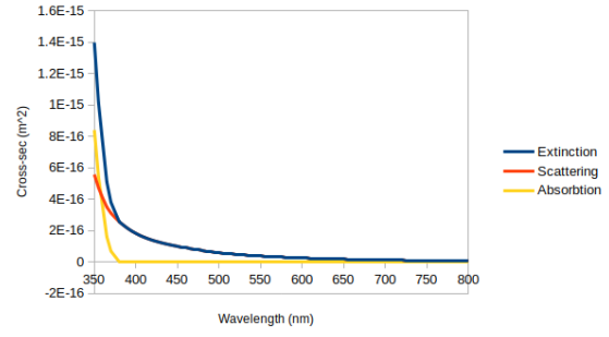
(b) 50 nm \text{TiO}_2 NP
