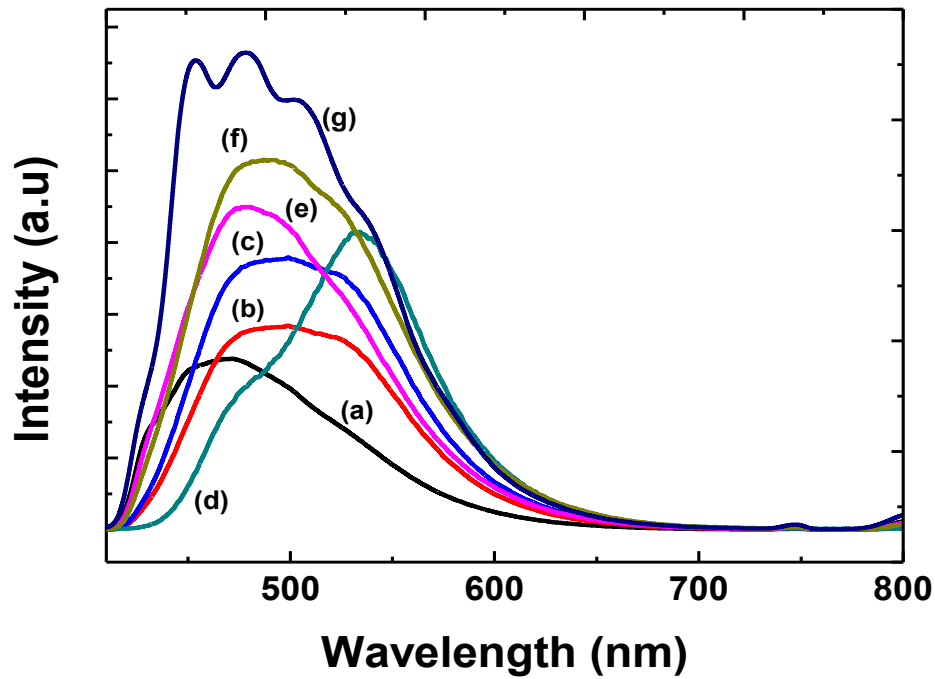
Figure 4.6: PL spectra of OLA/ \beta - \text{In}_2\text{S}_3 nanostructures at (a) 60 min, (b) 90 min, (c) 120 min, (d) 150 min, (e) 210 min, (f) 300 min, and (g) 330 min in the 1:1 (In:S) reaction system.
