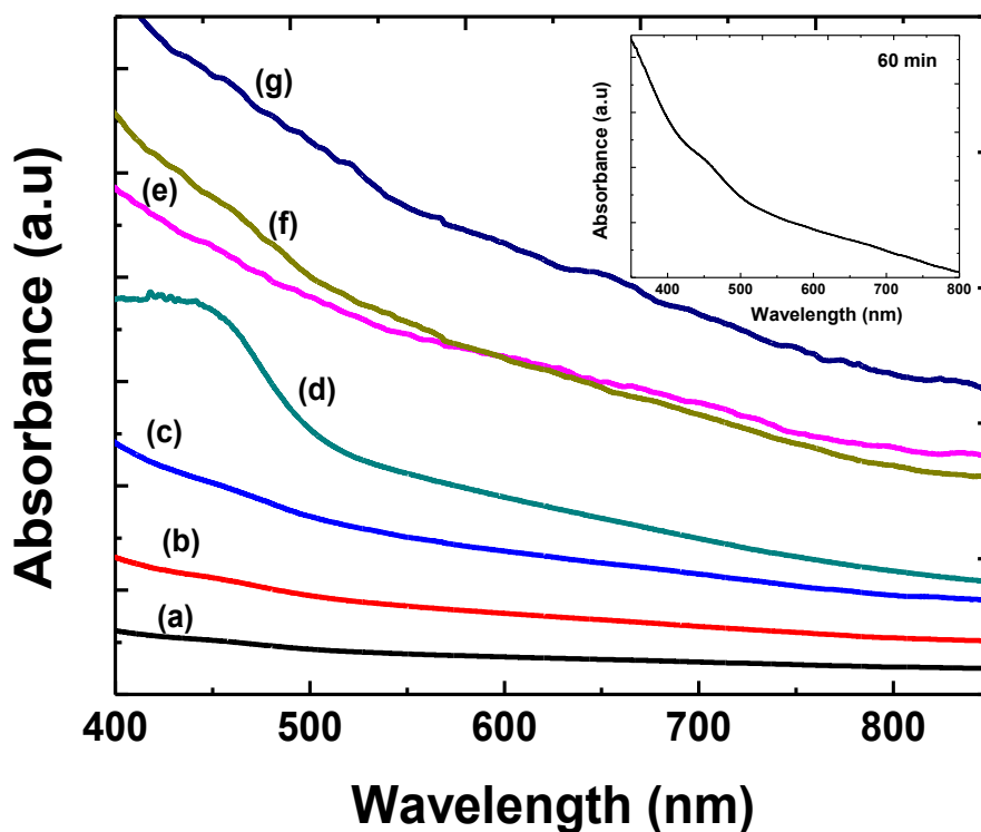
Figure 4.5: UV-vis spectra of OLA/ \beta - \text{In}_2\text{S}_3 nanostructures at (a) 60 min, (b) 90 min, (c) 120 min, (d) 150 min, (e) 210 min, (f) 300 min, and (g) 330 min in the 1:1 (In:S) reaction system.
