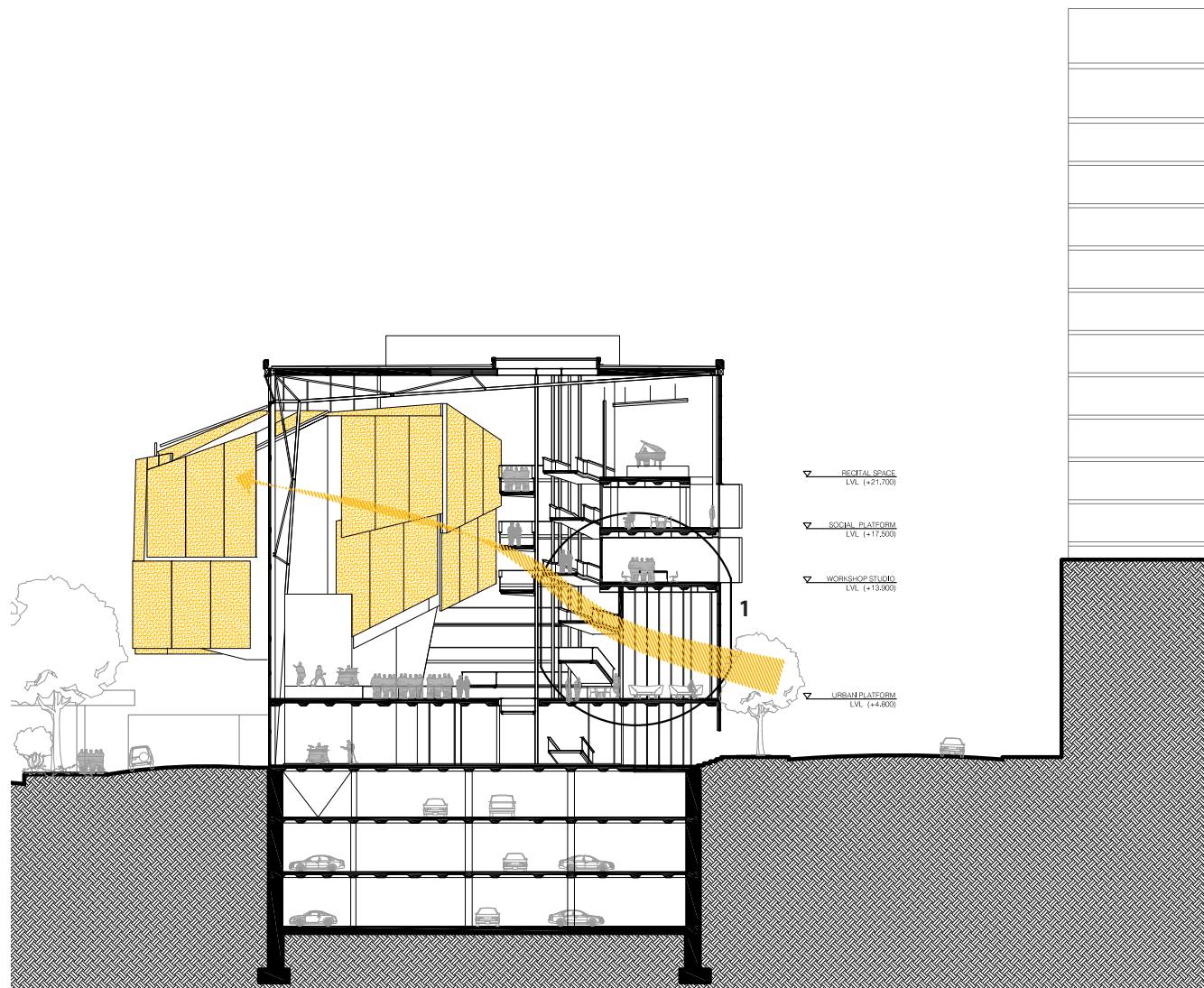
SECTION A-A
