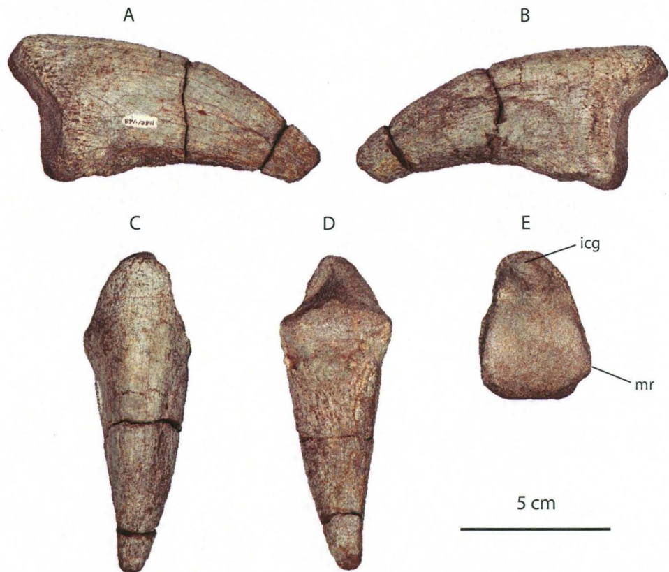
Figure 36: BP/1/7811, right pedal ungual. Lateral (A) medial (B) posterior (C) anterior (D) posterior (E). Abbreviations: icg, intercondylar groove; mr, medial ridge. Scale bar = 5 cm
