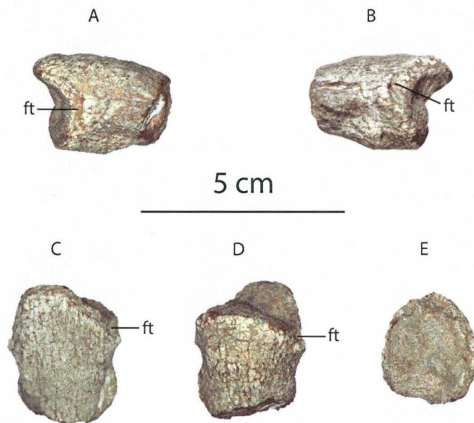
Figure 30: BP/1/7811 ?manual ungual phalanx. Lateral (A) medial (B) posterior (C) anterior (D) posterior (E). Abbreviations: ft, flexor tubercle. Scale bar = 5 cm.
