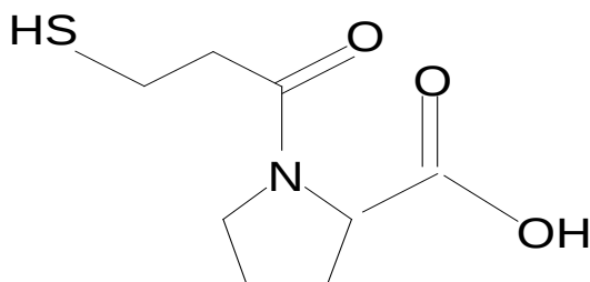
N-[(S)-3-Mercapto-2-methylpropionyl]-L-proline
