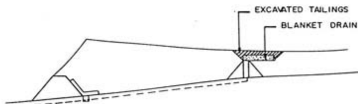
(d) ELEVATED BLANKET INSTALLED
