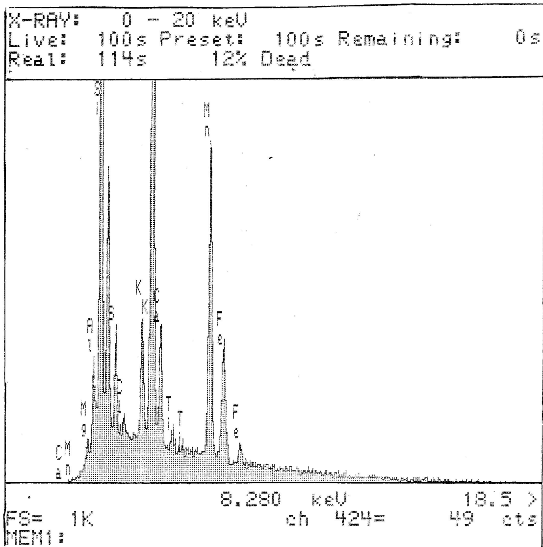
Figure 8.3.2 EDS Spectra II: Gypsum. Granular area.
