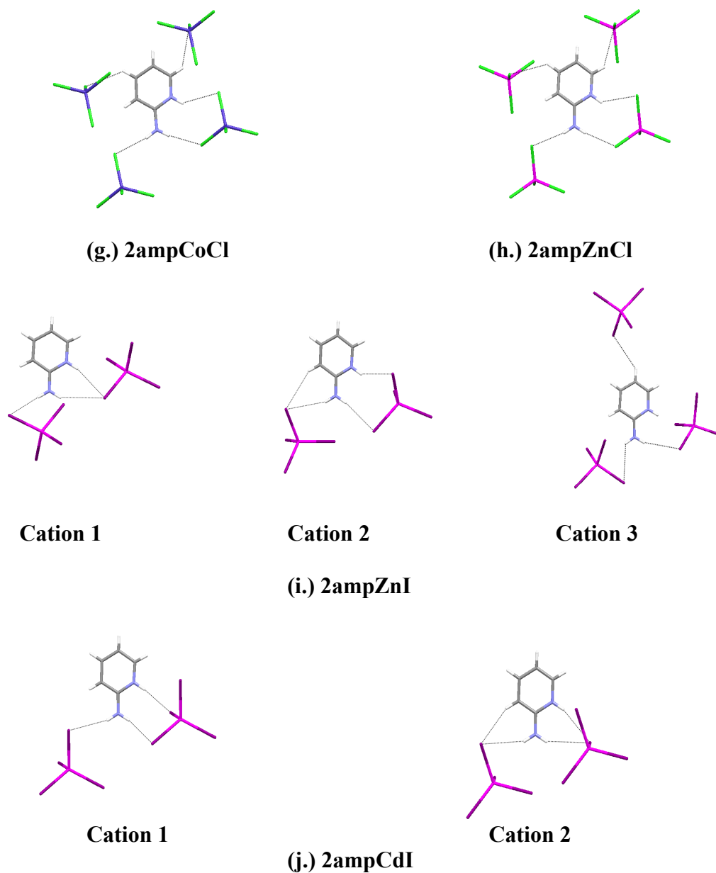
Figure 42: Identified synthons in (a.) 2ampHgCl. (b.) 2ampZnBr. (c.) 2ampCuCl (Kumar et al , 2005; YAPNAS01). (d.) 2ampCuBr (Luque et al , 1997; RIPWIW). (e.) 2ampHgI. (f.) 2ampHgBr. (g.) 2ampCoCl (Jebas et al , 2006; DELPOA). (h.) 2ampZnCl. (i.) 2ampZnI. (j.) 2ampCdI.
