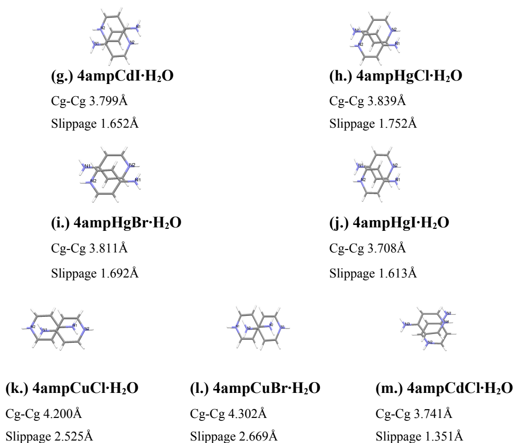
Figure 47: Cation pair orientation in (a.) 4ampZnCl, (b.) 4ampZnBr, (c.) 4ampZnI, (d.) 4ampCoCl (Jebas et al , 2009; HOSVIV), (e.) 4ampCdBr·H 2 O (Hatano et al , 2008; POGHEZ), (f.) 4ampCdBr·H 2 O (current study), (g.) 4ampCdI·H 2 O, (h.) 4ampHgCl·H 2 O, (i.) 4ampHgBr·H 2 O, (j.) 4ampHgI·H 2 O, (k.) 4ampCuCl·H 2 O (Halvorson et al , 1990; SEZLEO), (l.) 4ampCuBr·H 2 O (Román, 1996; ZUDKUE) and (m.) 4ampCdCl·H 2 O.
