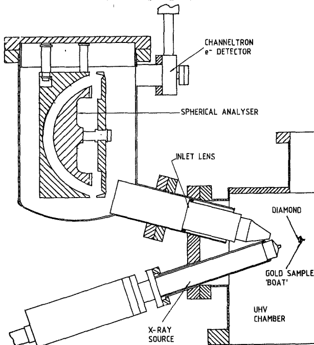
FIG. 18 XPS APPARATUS
