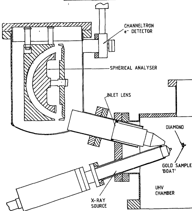
FIG. 18 XPS APPARATUS 15
