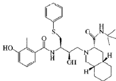
Nelfinavir
