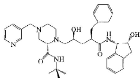
Indinavir
