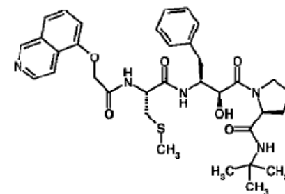
KNI-272
