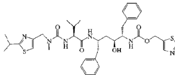
Ritonavir
