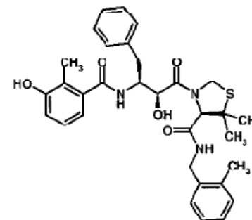
KNI-764
