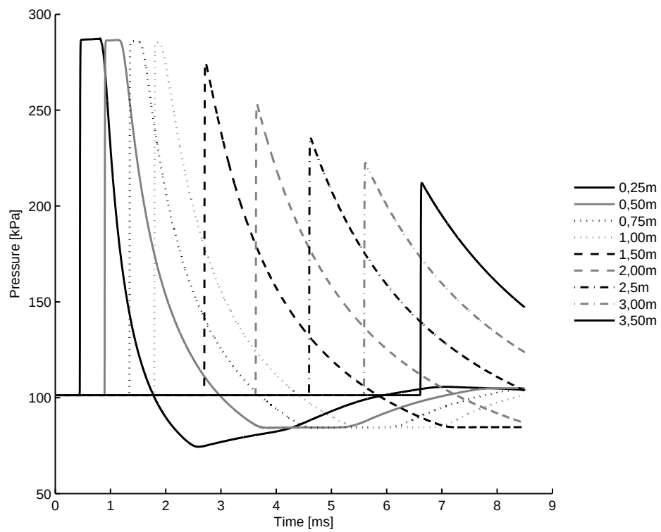
4.19 (d): 90mm 10bar
