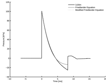
4.50 (d): Convex Profile 10bar 3.00m
