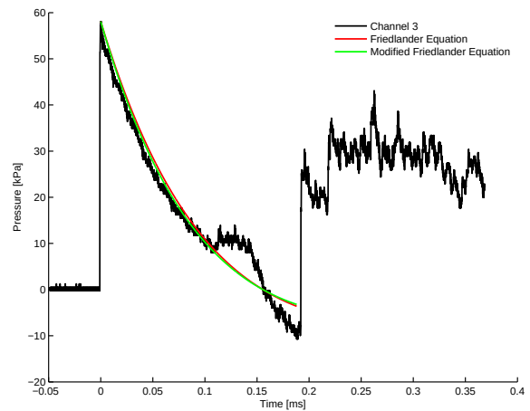
7.2 (d): Concave Profile 100\mu m \approx 1000kPa 2.98m
