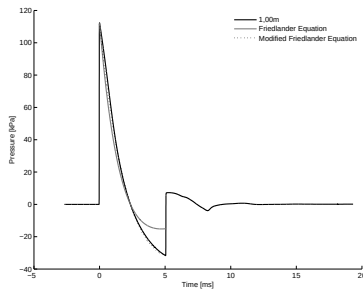
4.49 (b): Linear Profile 10\text{bar} 1.00\text{m}
