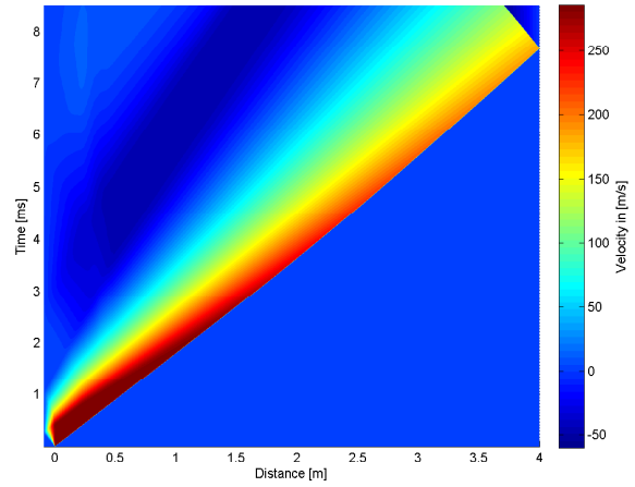
4.24 (d): 90mm 10bar
