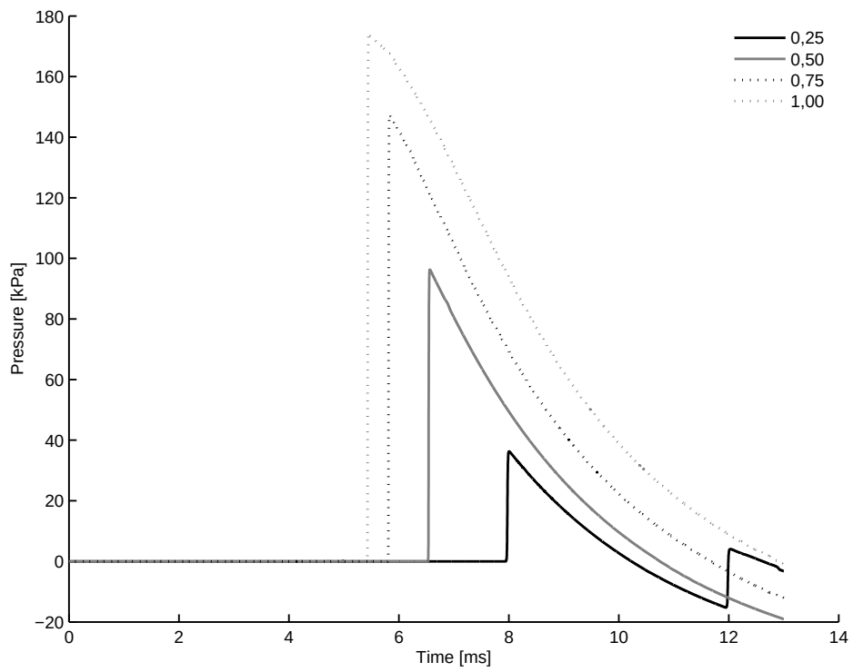
4.32 (d): 3.00m 10bar
