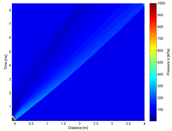
4.9 (d): 45^\circ 10bar
