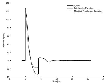
4.49 (a): Linear Profile 10\text{bar} 0.25\text{m}
