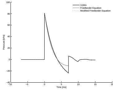
4.49 (d): Linear Profile 10bar 3.00m
