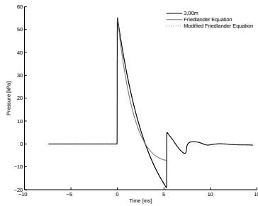
4.48 (d): Concave Profile 10\text{bar} 3.00\text{m}
