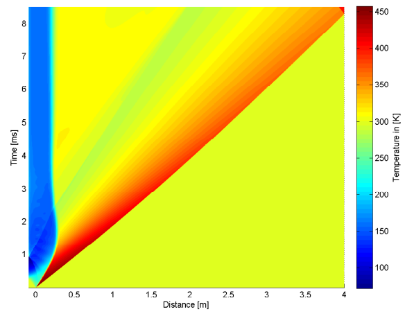
4.11 (d): 45^\circ 10bar
