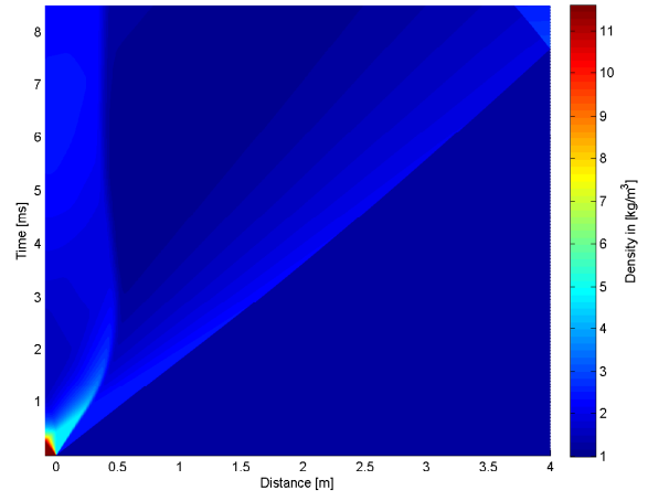
4.22 (d): 90mm 10bar
