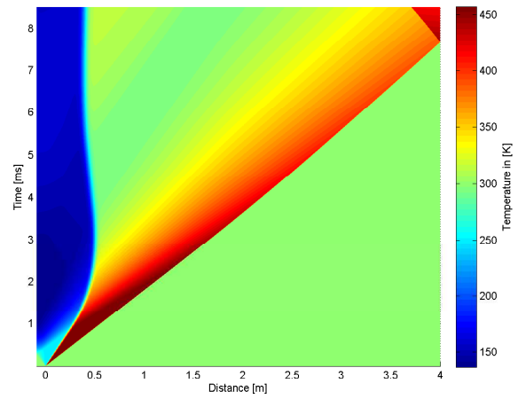
4.23 (d): 90mm 10bar
