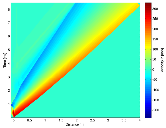
4.12 (d): 45^\circ 10bar
