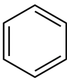
(ii) benzene
