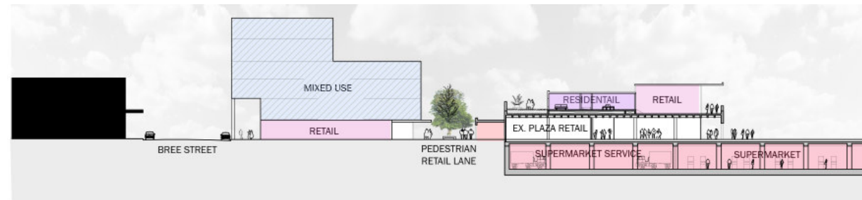
SECTION D-D 1:1000
