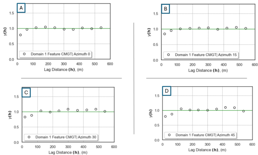
Figure B4: Experimental variograms a) Domain 1 Au (cm.g/t) azimuth 0 b) Domain 1 Au (cm.g/t) azimuth 15 c) Domain 1 Au (cm.g/t) azimuth 30 d) Domain 1 Au (cm.g/t) azimuth 45.
