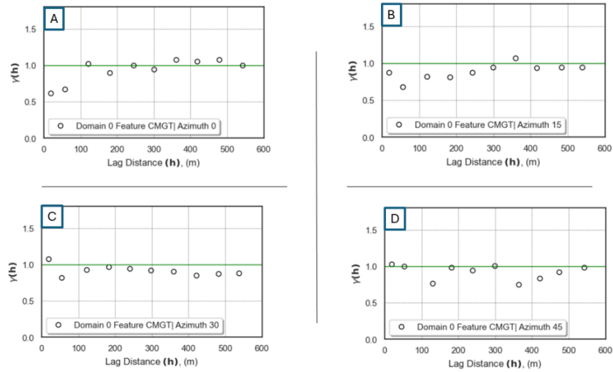
Figure B1: Experimental variograms a) Domain 0 Au (cm.g/t) Azimuth 0 b) Domain 0 Au (cm.g/t) Azimuth 15 c) Domain 0 Au (cm.g/t) Azimuth 30 d) Domain 0 Au (cm.g/t) Azimuth 45.
