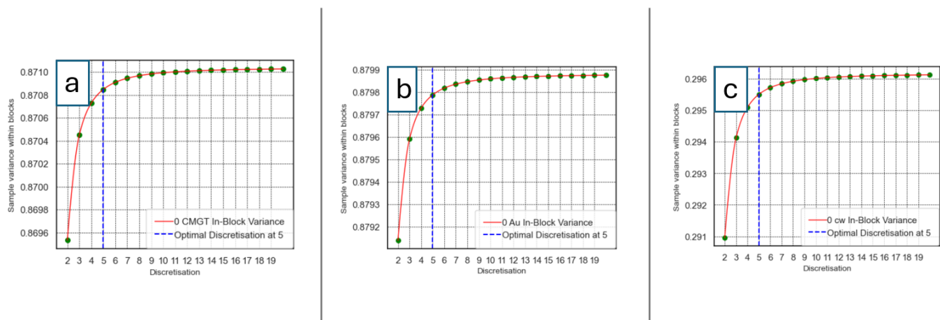
Figure 4.42: Block discretisation a) Domain 0 Au (cm.g/t) b) Domain 0 Au (g/t) c) Domain 0 CW (cm).
