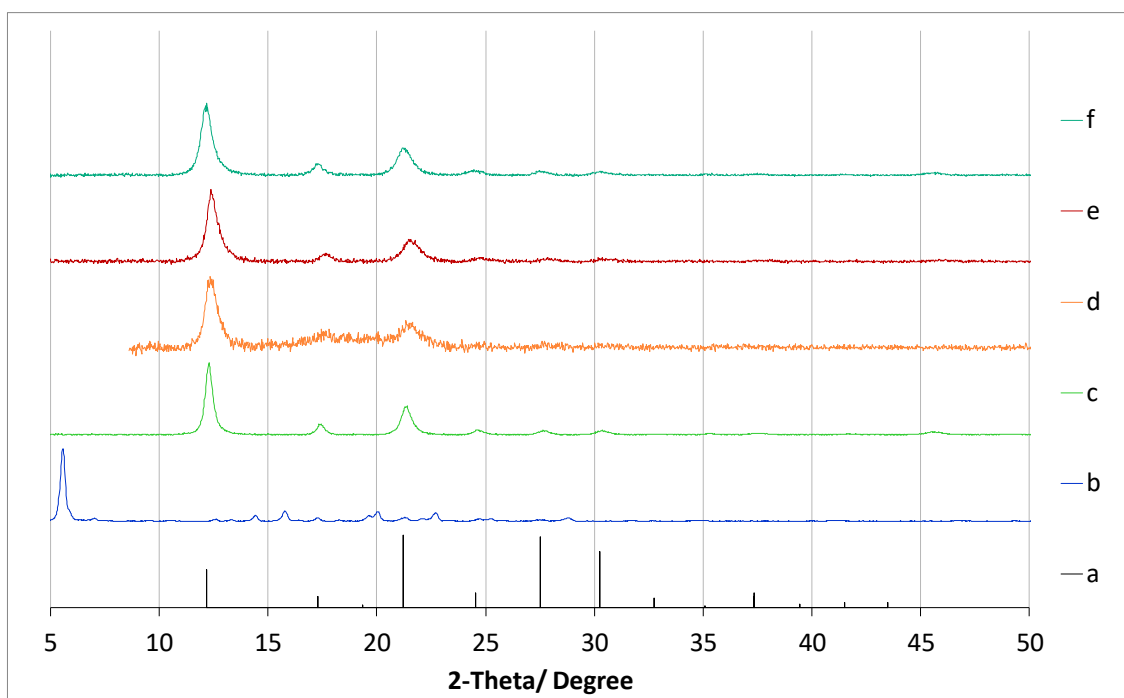
Figure 28: XRD patterns for a) simulated IZA standard; b) RUB-15 (MMM); c) SSOD m; d) OPT 1; e) OPT 2; f) OPT 3
