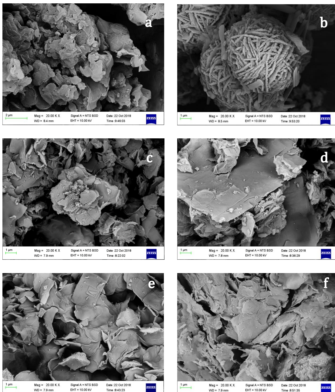
Figure A: SEM imaging for synthesized samples a)RUB-15; b)HSOD; c)SSOD1; d)SSOD2; e)SSOD3; f)SSOD4; g)SSOD5; h)SSOD6; i)SSOD7; j)SSOD8; k)SSOD9
