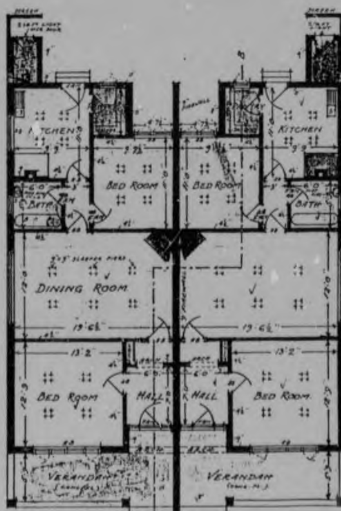
PLAN.
