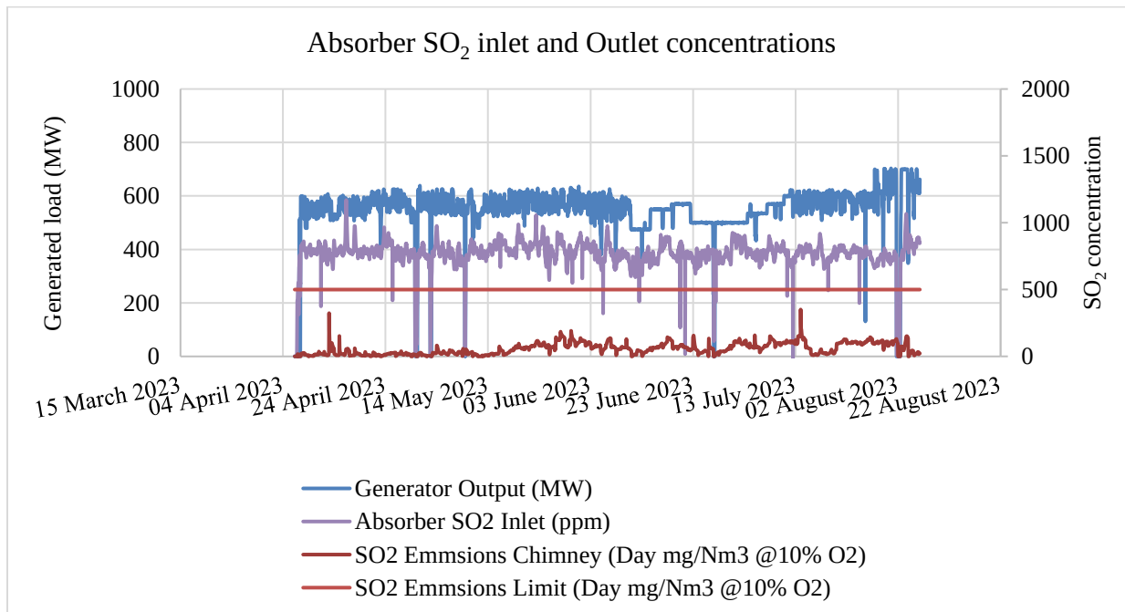
Figure 4.2.1.6-1: Actual SO 2 emissions
