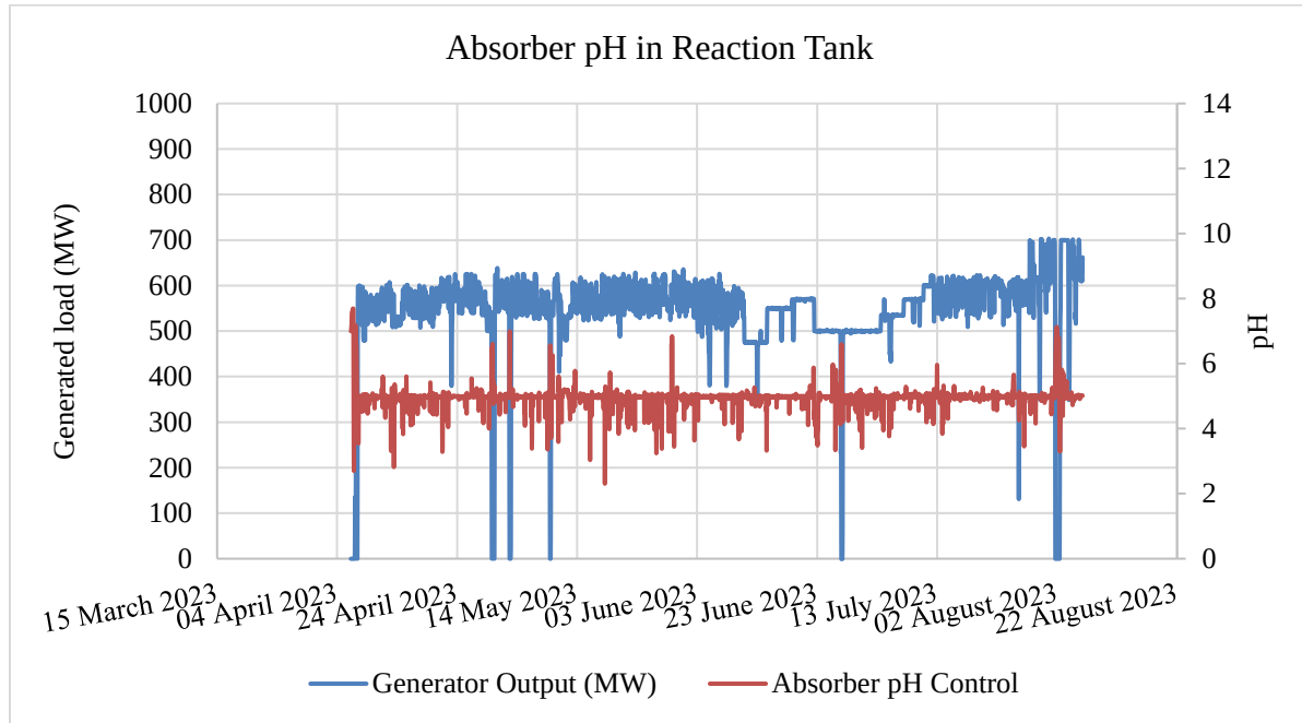
Figure 4.2.1.3-1: Actual absorber pH
