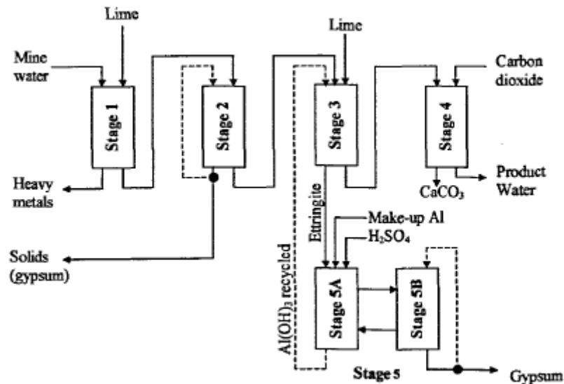
Figure 2. 16 SAVMIN process (Van Niekerk, 2002)
