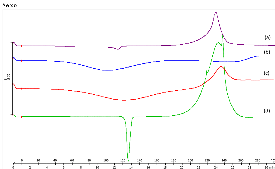
Figure 4.8: DSC thermograms of; (a) PEC-MUC-PEG +AZT, (b) MUC, (c) PEC and (d) AZT
