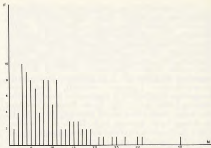
Figure 5. Australoxylon natalense nov. gen. n. sp., Histogramme montrant la variation du nombre des cellules couchées formant la hauteur des rayons. (F): fréquence. (N): nombre de cellules.
