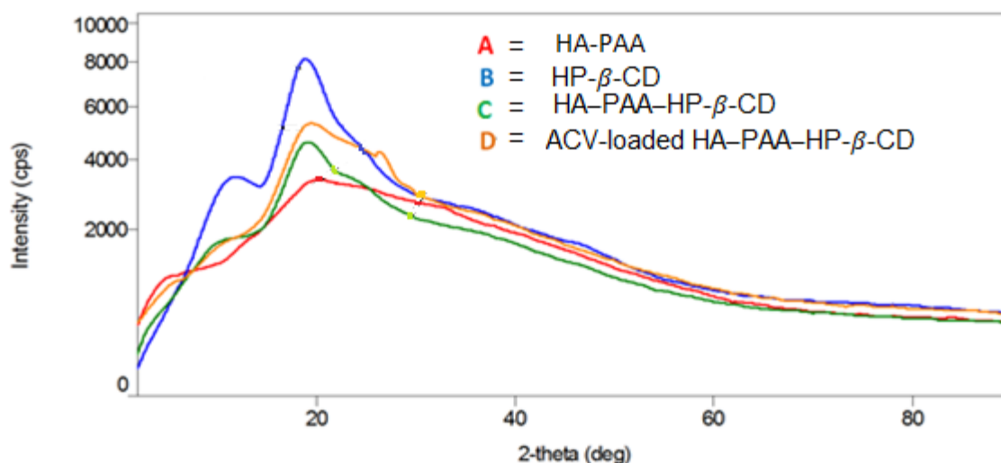
Figure 3.7: The XRD spectra for (a) HA–PAA, (b) HP-β-CD, (c) HA–PAA–HP-β-CD and (d) ACV-loaded HA–PAA–HP-β-CD.
