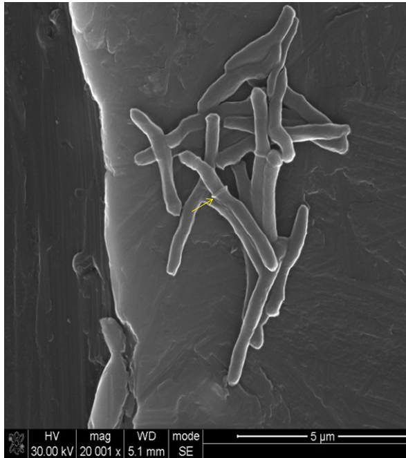
\Delta rpfB
