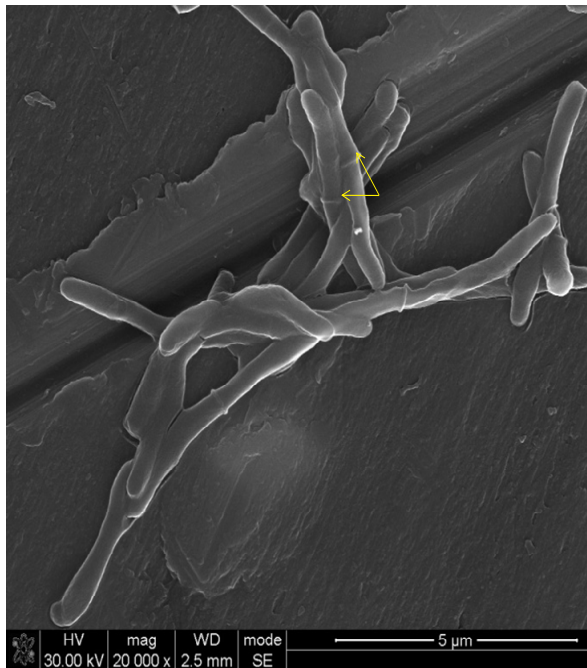
\Delta rpfB
