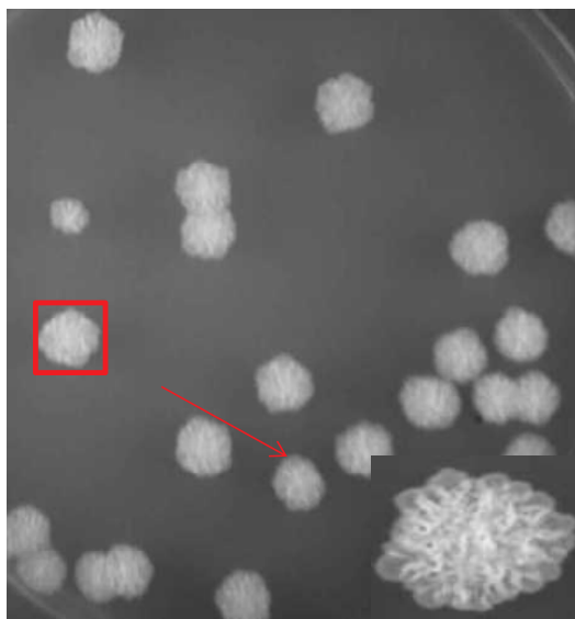
\Delta rpfB
