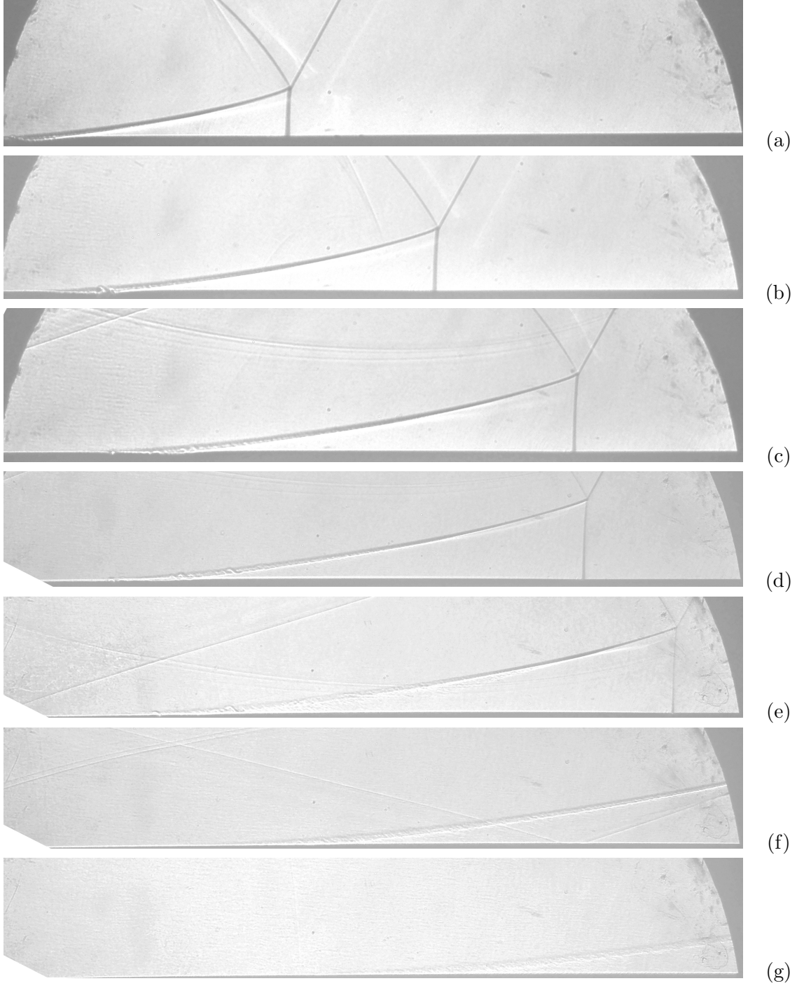
Figure 6.1: Shear layer development for the 30° Wedge. M_s = 1.37 . (a) 3100\mu s , (b) 3200\mu s , (c) 3300\mu s , (d) 3350\mu s , (e) 3400\mu s , (f) 3600\mu s , (g) 3800\mu s
